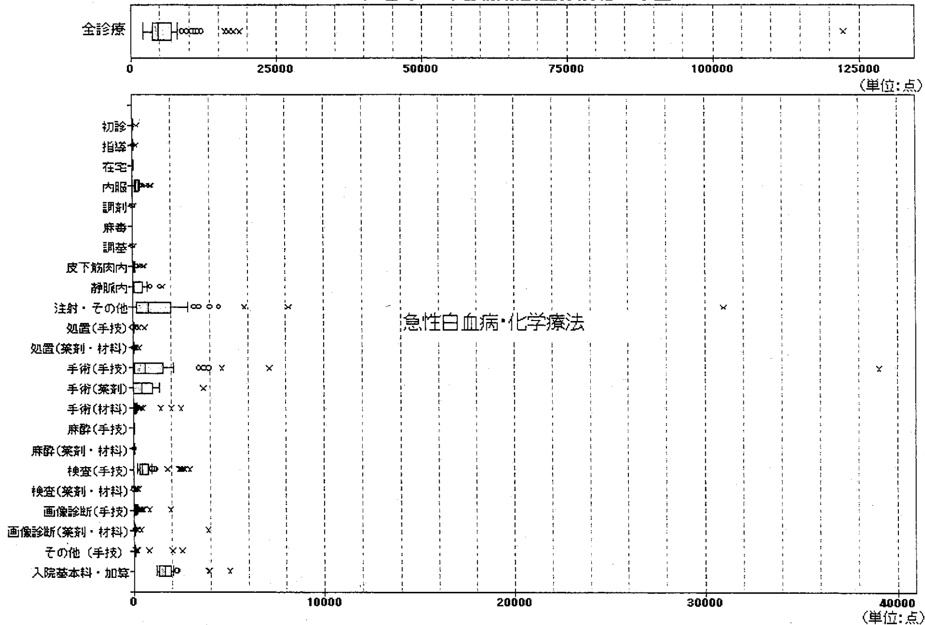
(1日あたり)診療報酬区分別箱ひげ図
