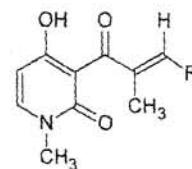
エフロトマイシン A 1 (E isomer)
